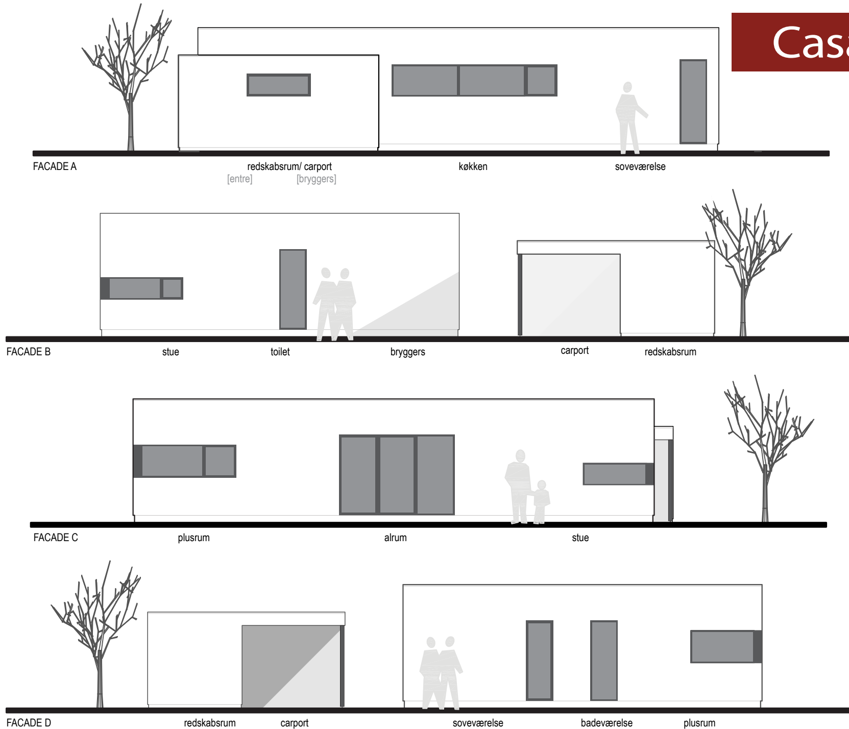
CasaBo type csb1 • carport • spejlvendt model • 1:100
